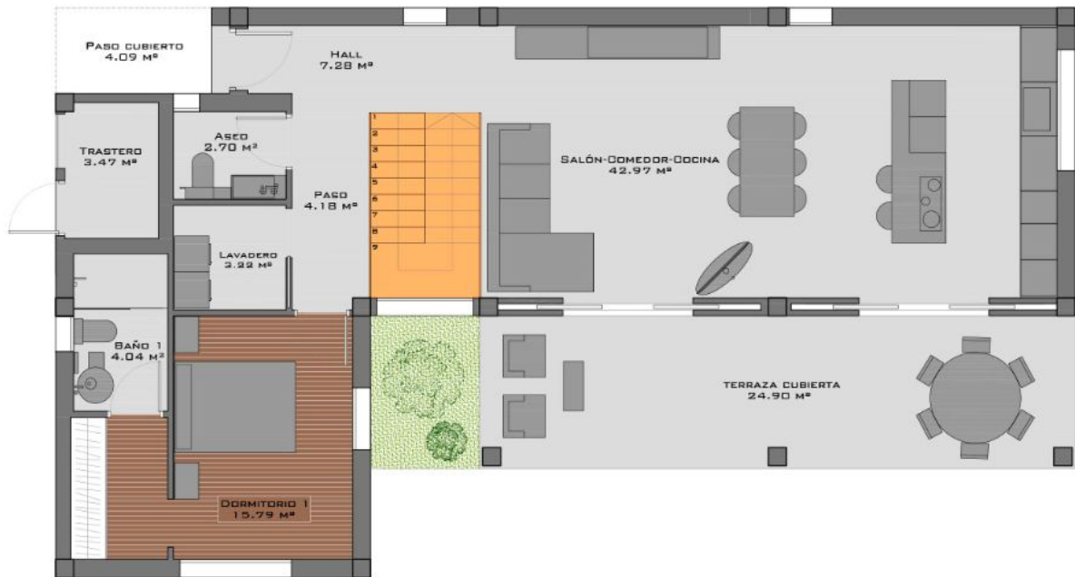
Nedre plan - exempel med öppet kök
